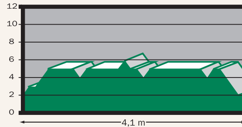
Abonadora HIO
